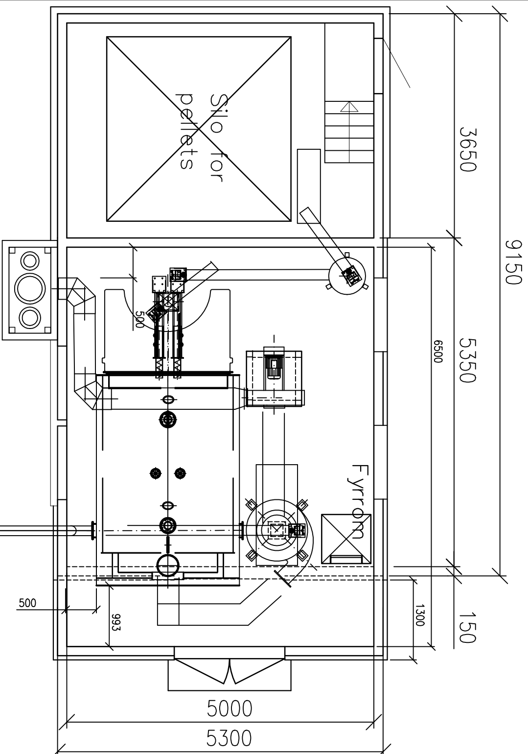
Plan 1. etasje
